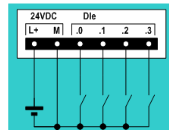
6ES7 221-3BD30-0XB0
