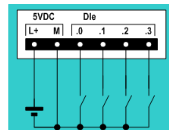
6ES7 221-3AD30-0XB0
